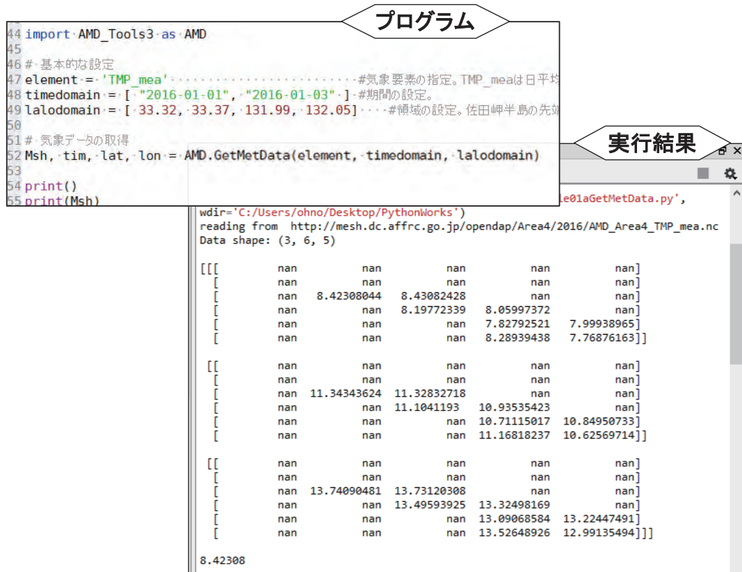
図 IV-1. サンプルプログラム sample_GetMetData-a.py の 44 行～ 55 行目（左上）と対応する実行結果（右下）
