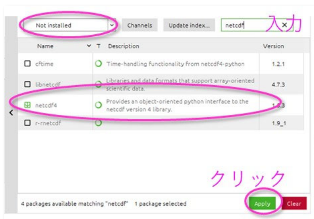
図6. Anaconda Navigator の「Environments」メニューで「Not installed」を選択し、インストールしたいモジュール名を検索枠に入力。
