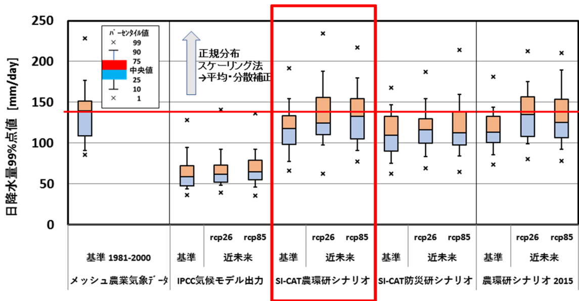
図2 図1に同じ、ただし高知市付近における日降水量年間99パーセントイル値を示す（出典同）。
